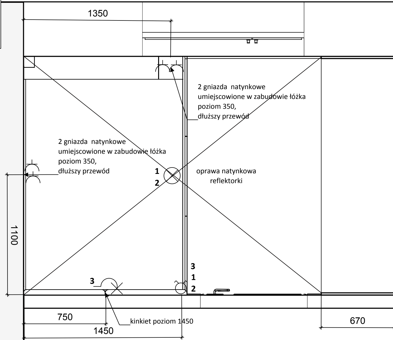
SYPIALNIA - UKŁAD ELEKTRYCZNY
